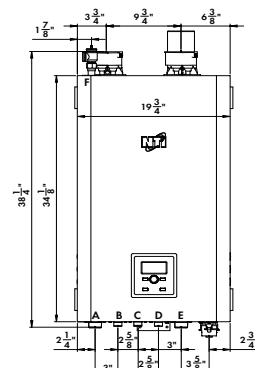
TRX150, 199, 199C
